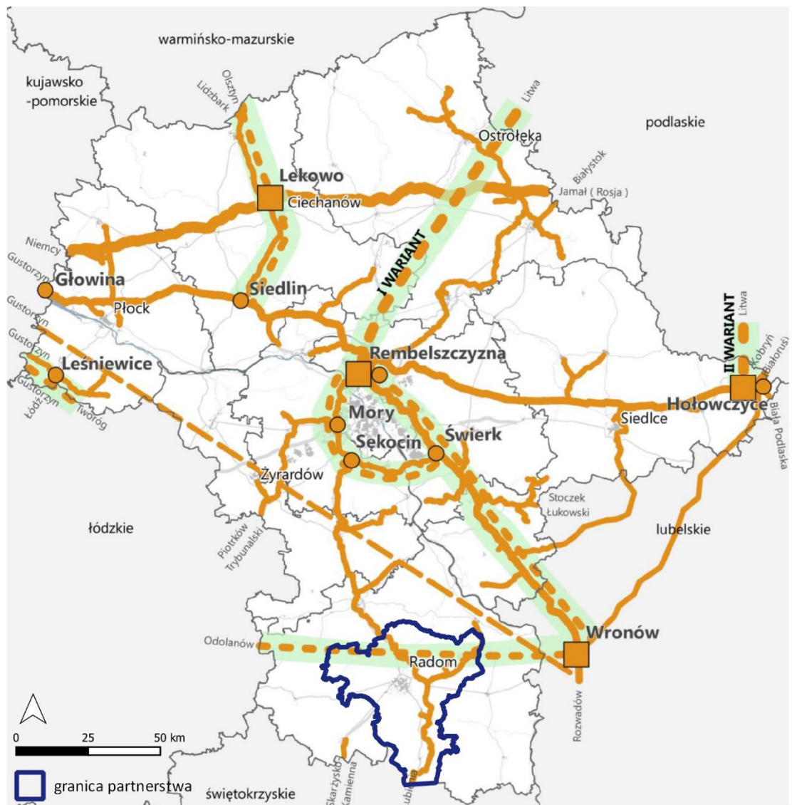
Ryc. 66 System gazowy wysokiego ciśnienia w województwie mazowieckim
