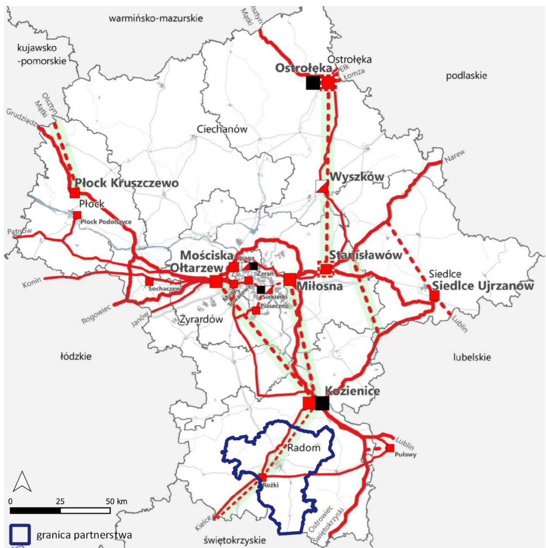
Ryc. 65. System elektroenergetyczny najwyższych napięć w województwie mazowieckim
